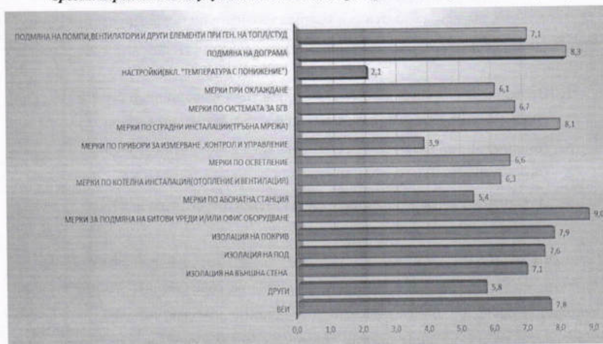
Средни периоди на откупуване на най-често препоръчвани енергоспестяващи мерки
